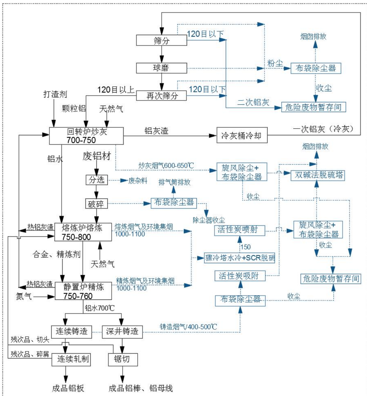
图 3.3-1 项目再生铝生产铝棒、铝板工艺流程及产污环节图
