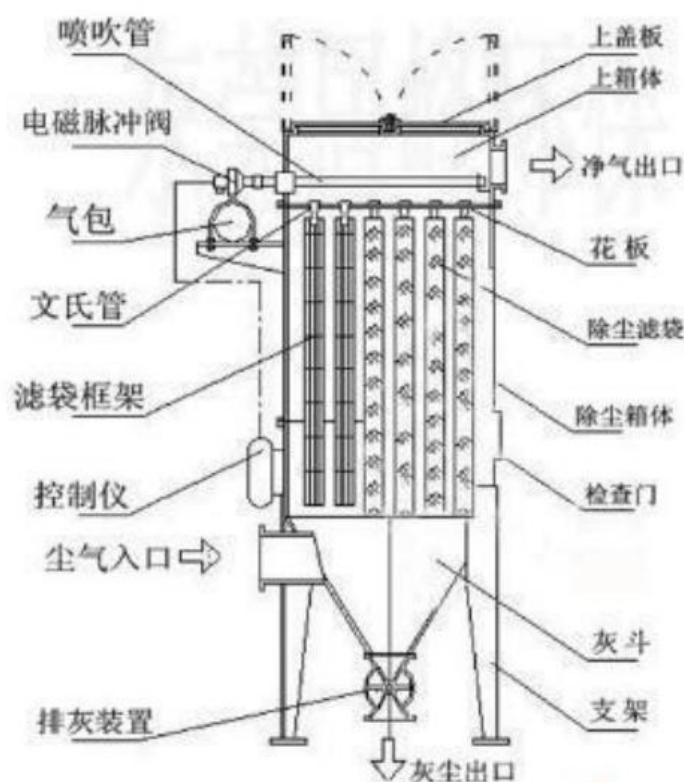
图 7.2-1 布袋除尘器结构示意图
