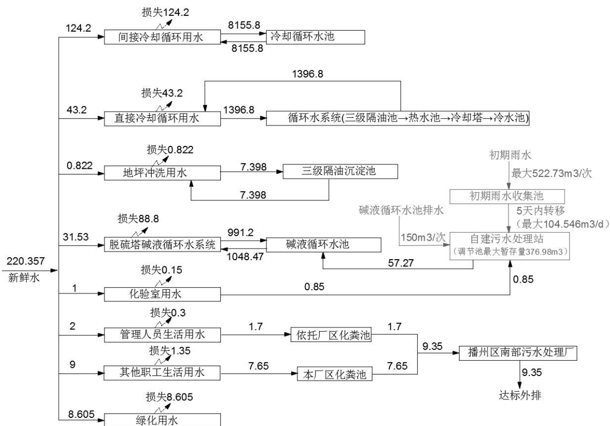
图 3.1-1 项目全厂水平衡图 (单位: \text{m}^3/\text{d} )
