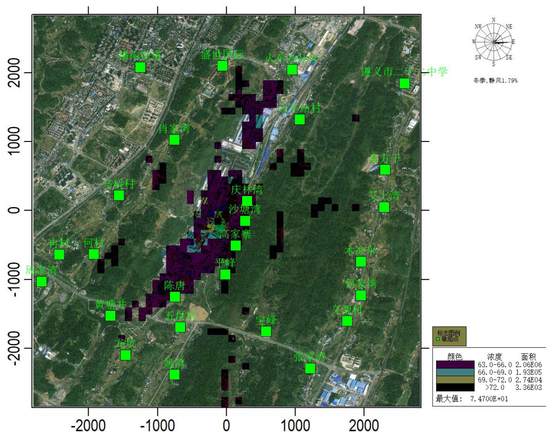
图 5.4.3-6 背景值叠加后 PM 10 日平均质量浓度分布图 (单位: \mu\text{g}/\text{m}^3 )
