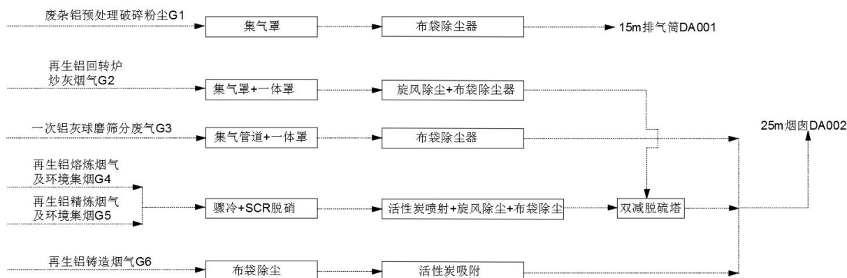
图 3.4-1 本项目废气污染防治及排放系统图
