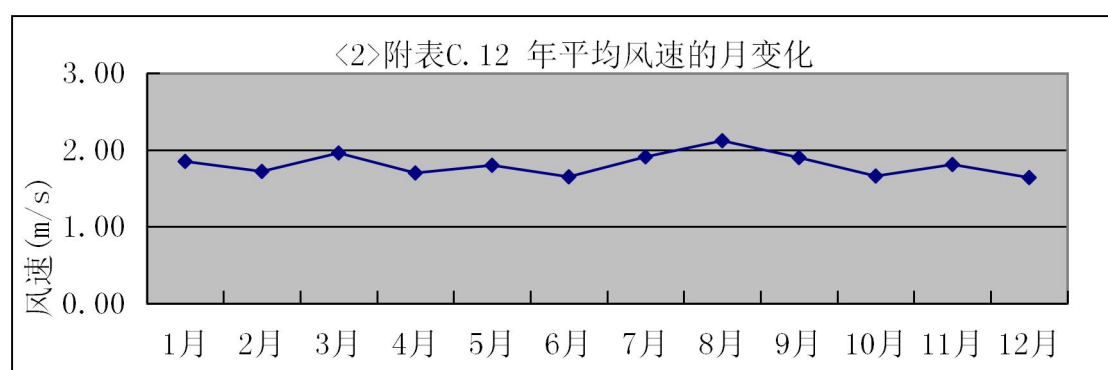
图 5.4-3 年平均风速的月变化图
