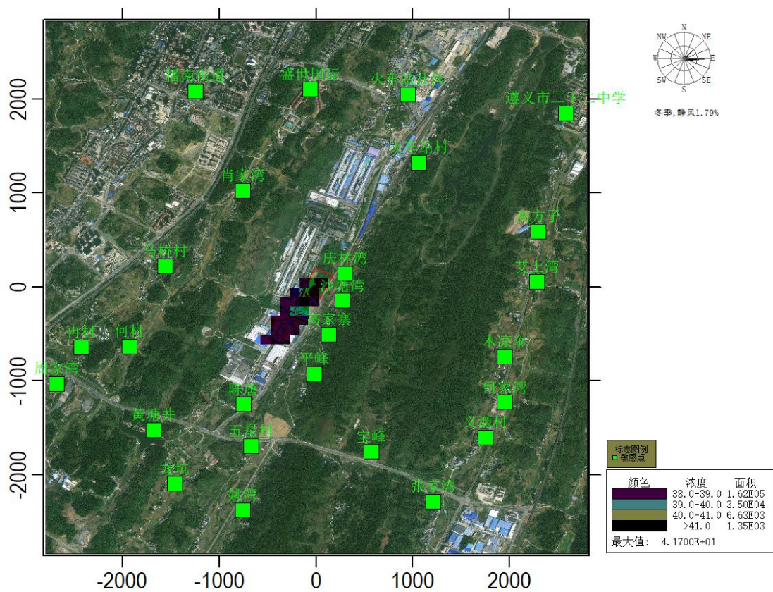
图 5.4.3-7 背景值叠加后 PM 10 年平均质量浓度分布图 (单位: \mu\text{g}/\text{m}^3 )
